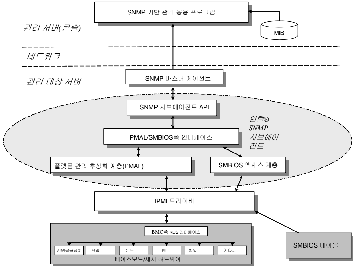
그림 1. 인텔® SNMP 서버에이전트 아키텍처
