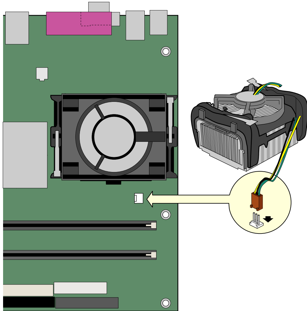
图 5. 将处理器风扇散热器电缆连接到处理器风扇连接器上
