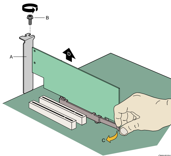
图 7. 拆卸 AGP 卡
