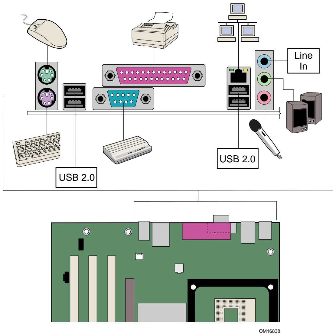
图 13. 背面板连接器
