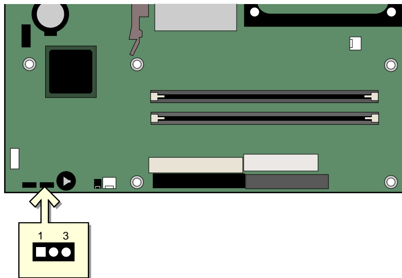
图 12. BIOS 配置跳线块的位置
