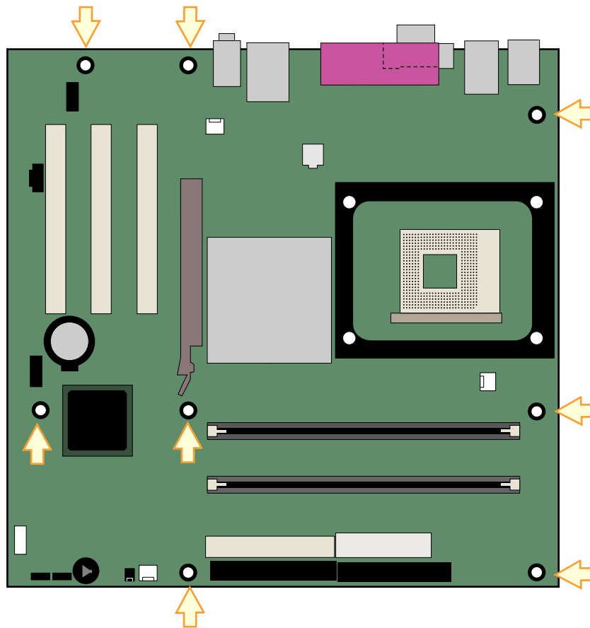
图 3. 安装螺丝孔位置
