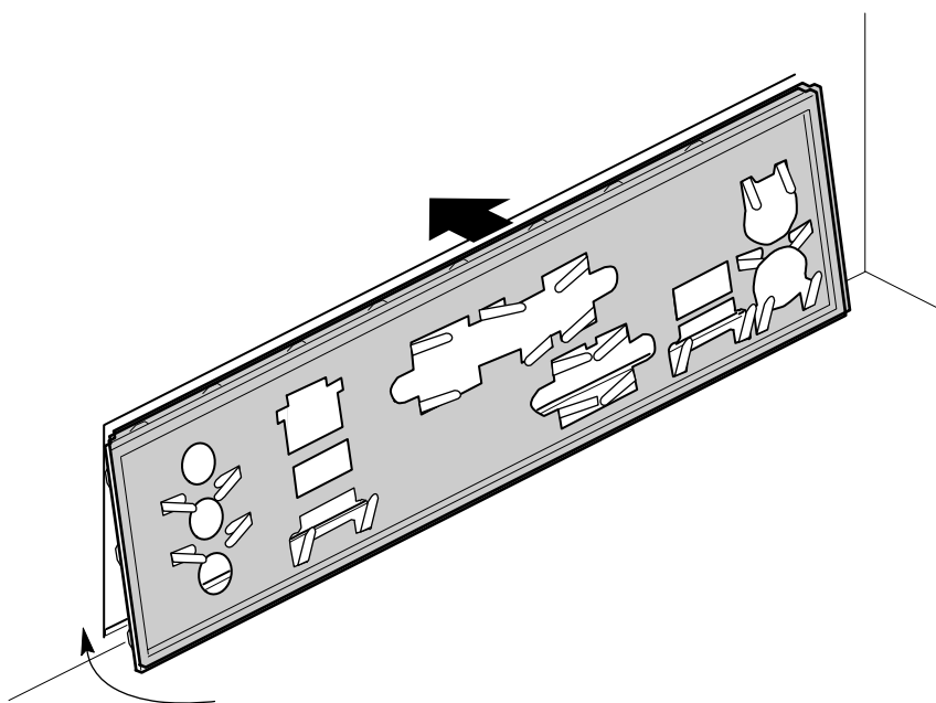
图 2. 安装 I/O 防护板
