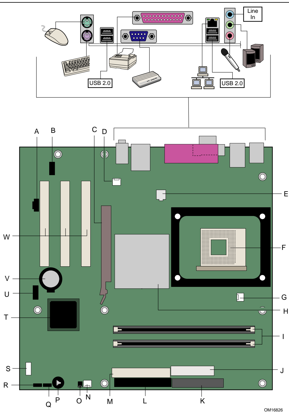
图 1. 桌面主板 D865PCD 组件
