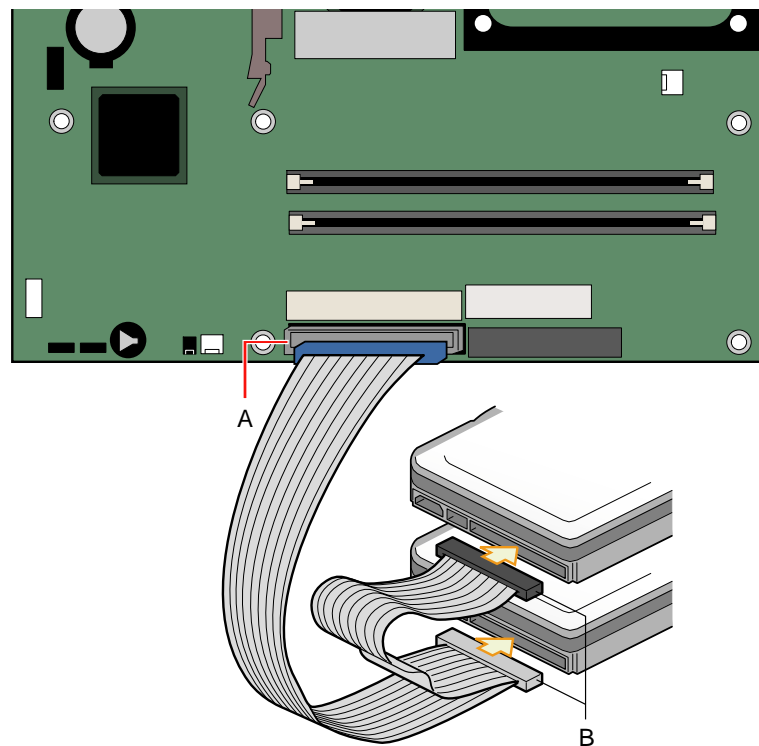
图 8. 连接 IDE 电缆
