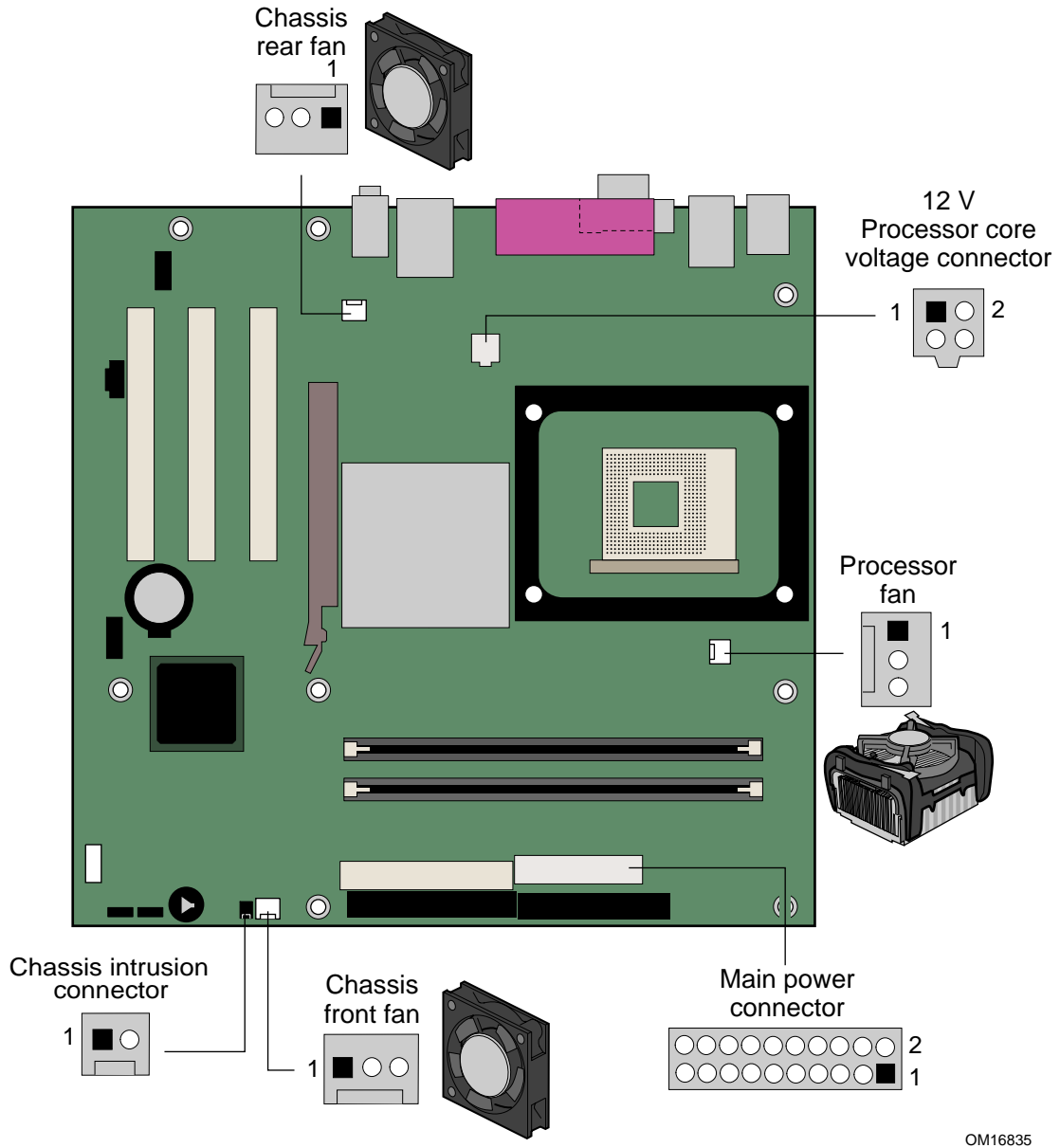
图 10. 硬件控制接头连接器和电源系统连接器的位置
