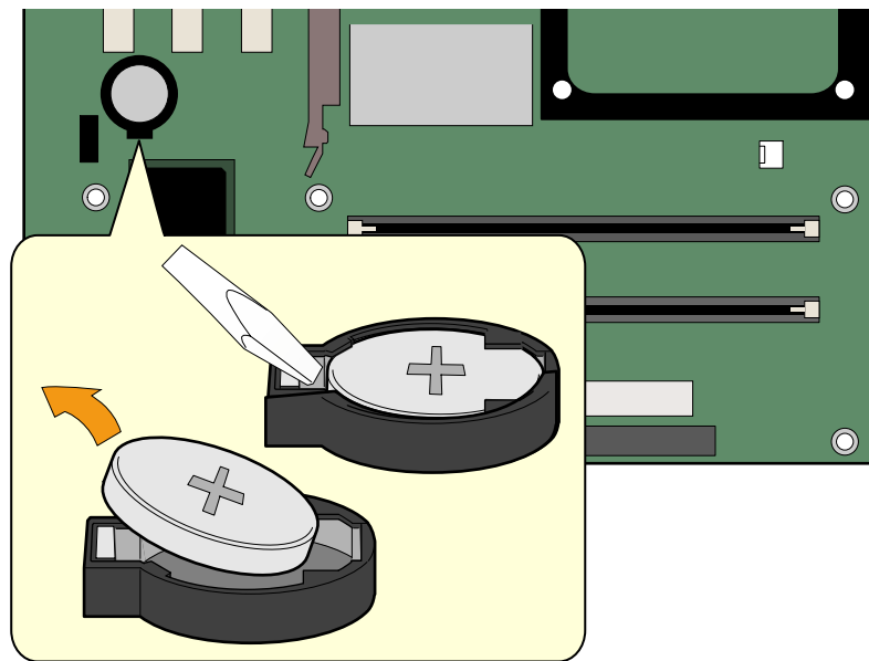
图 14. 拆卸电池
